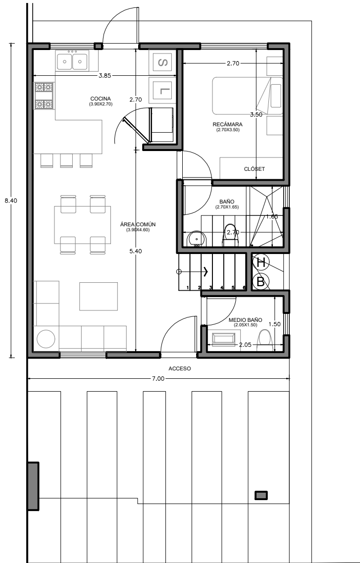
PLANTA BAJA
