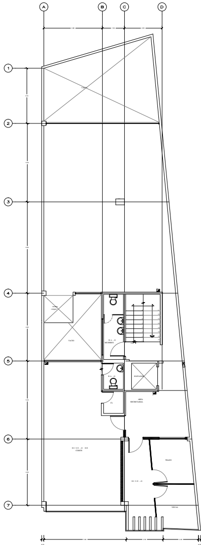
TERCER NIVEL
