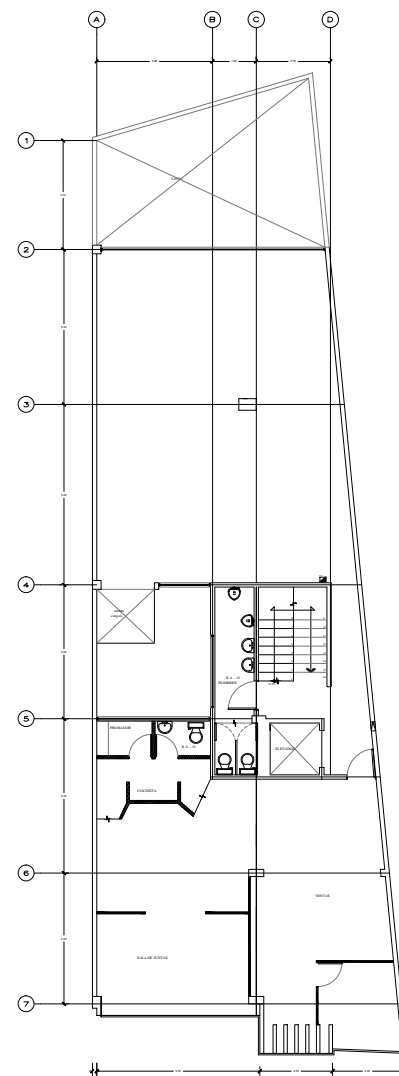
SEGUNDO NIVEL
