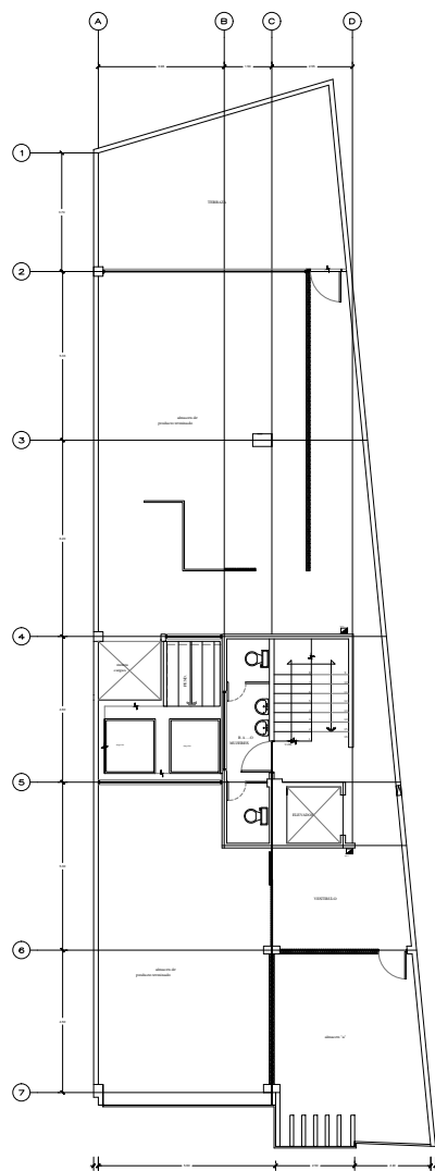
PRIMER NIVEL
