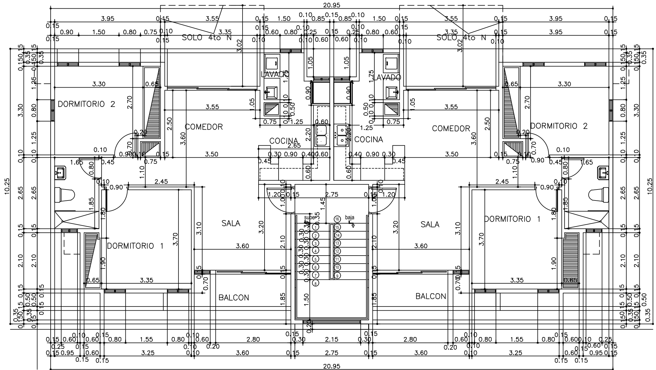
PLANTA DIMENSIONADA 2do y 3er N (BLOQUES .....)
