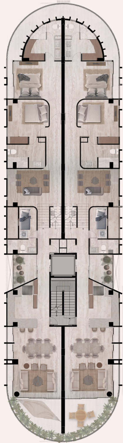
PLANTA BAJA
