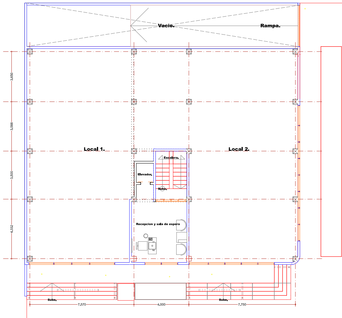
Planta Baja.
