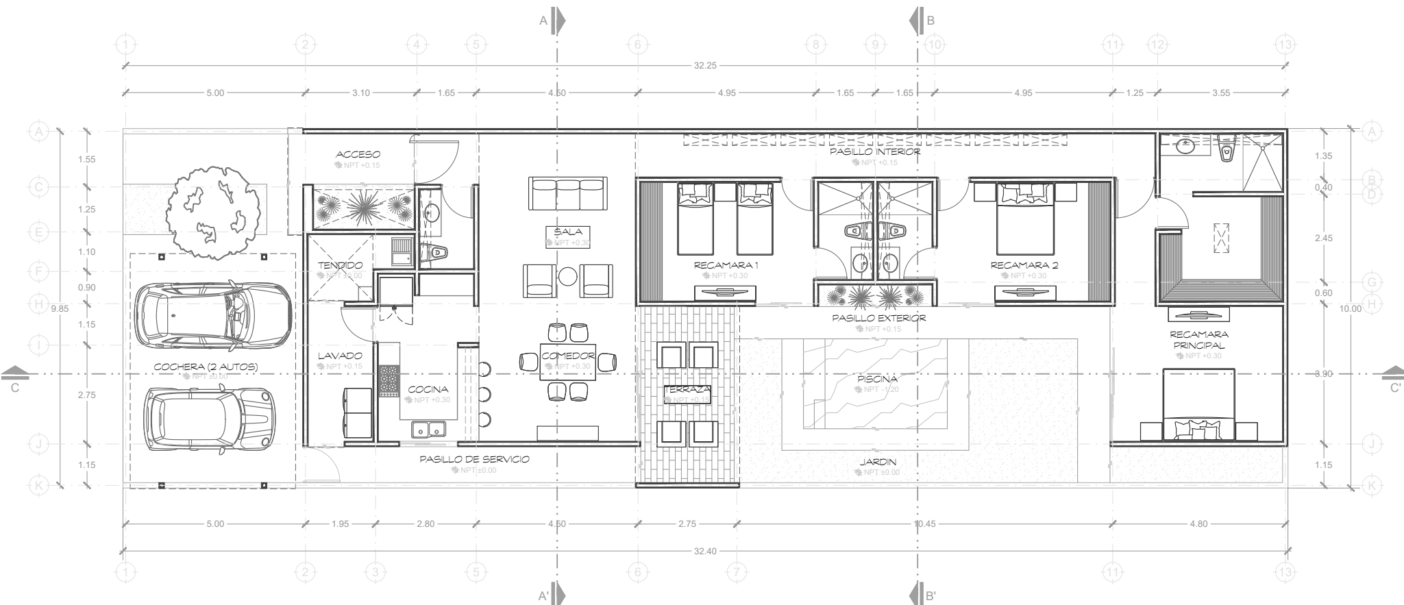
PLANTA ARQUITECTONICA
