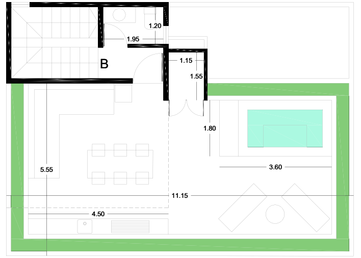
ROOFTOP DISTRIBUCIÓN
