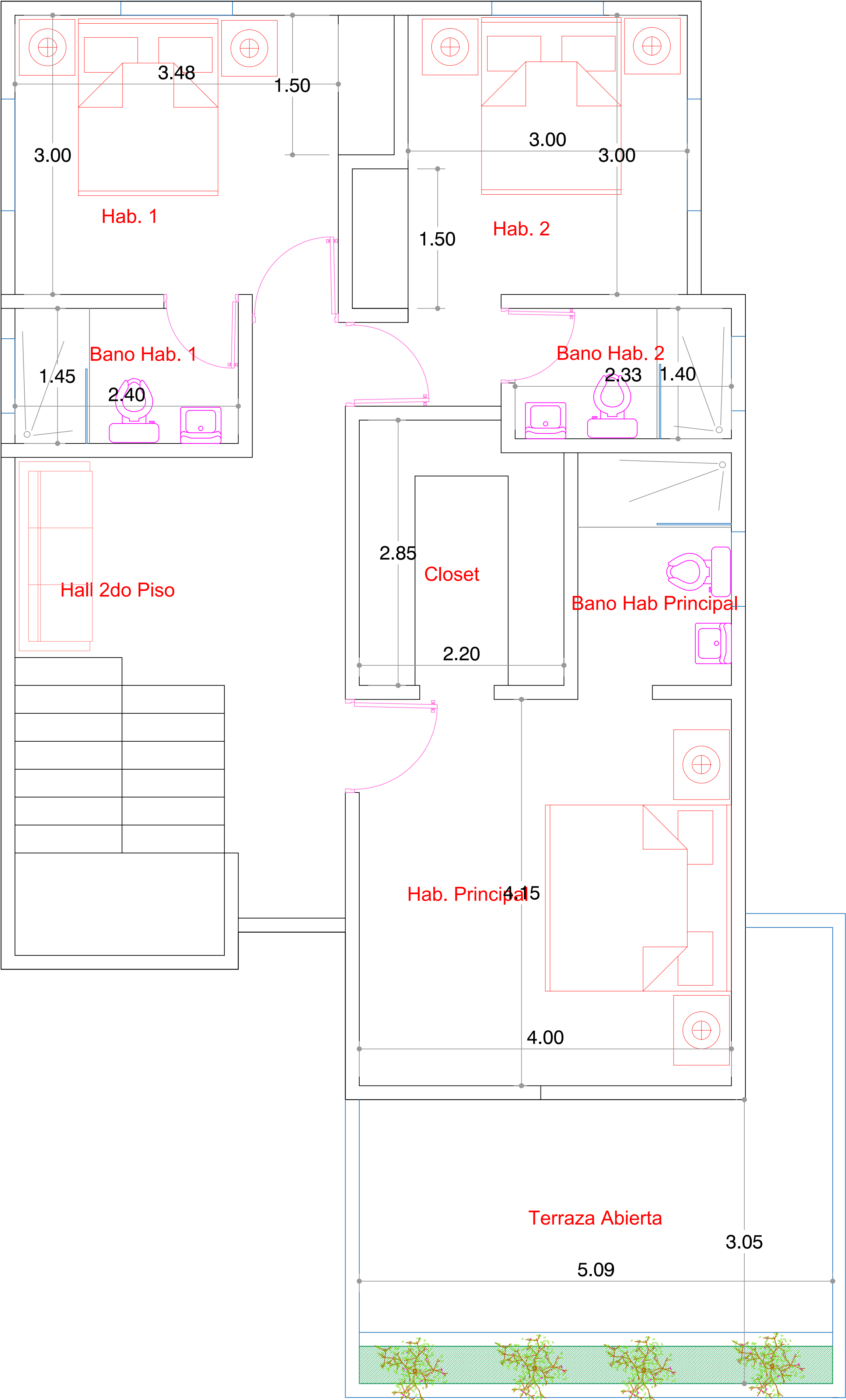
Planta Arquitectonica 2do Nivel
