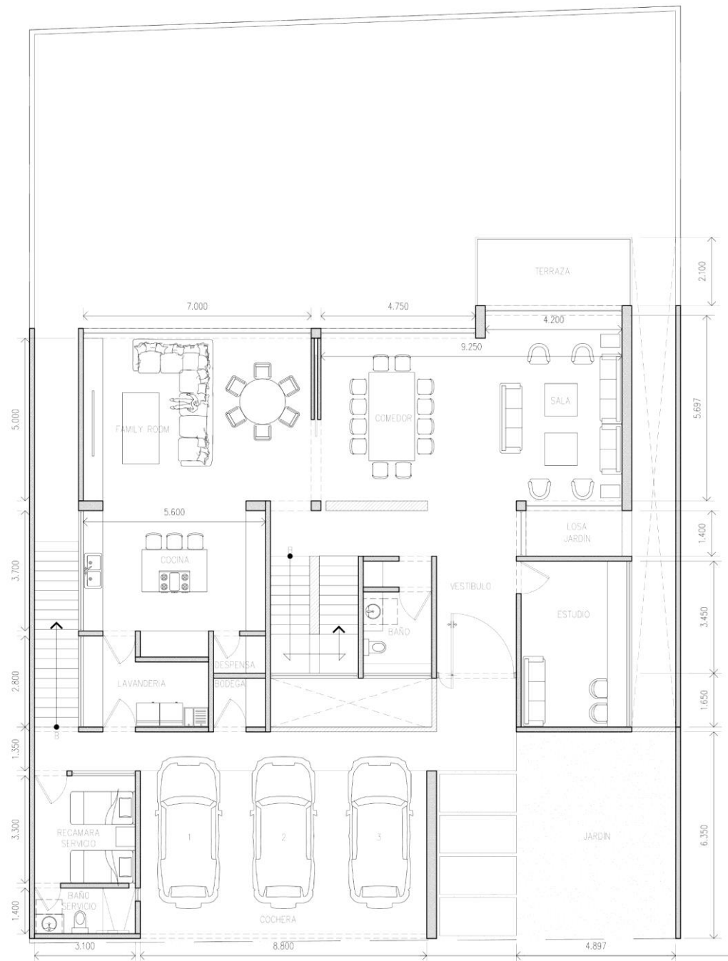
PLANTA BAJA
