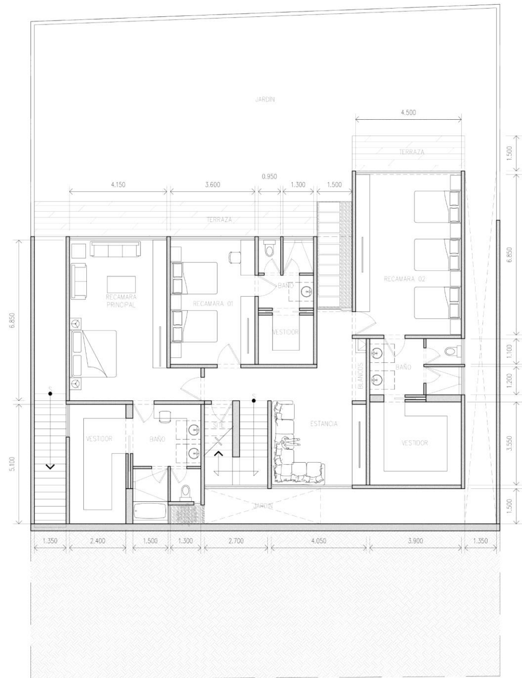
PLANTA SOTANO
