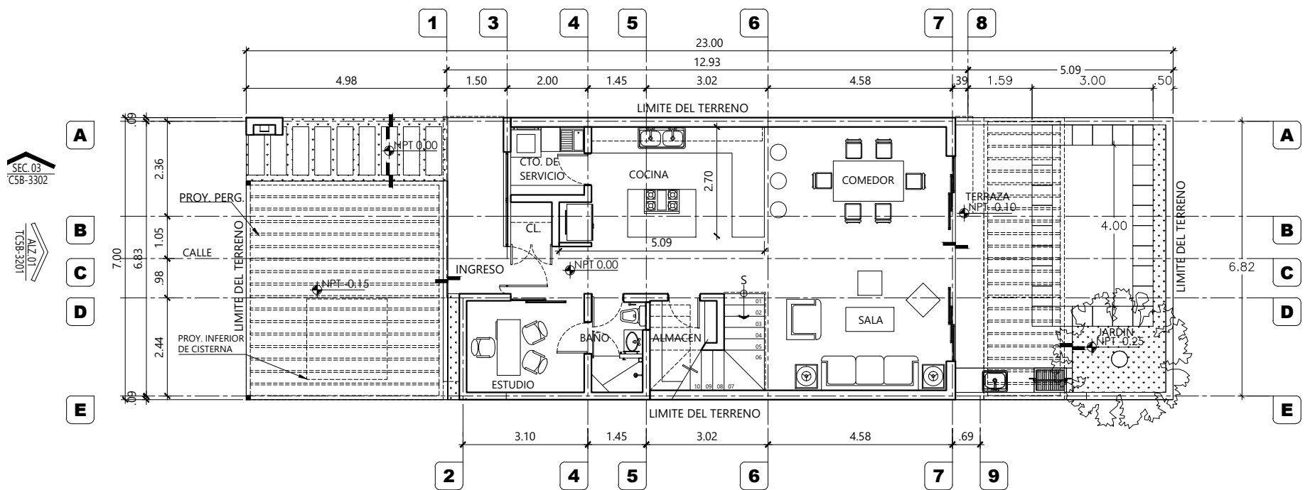
Planta Baja
