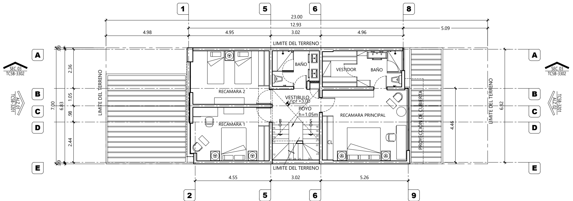
Planta Alta
