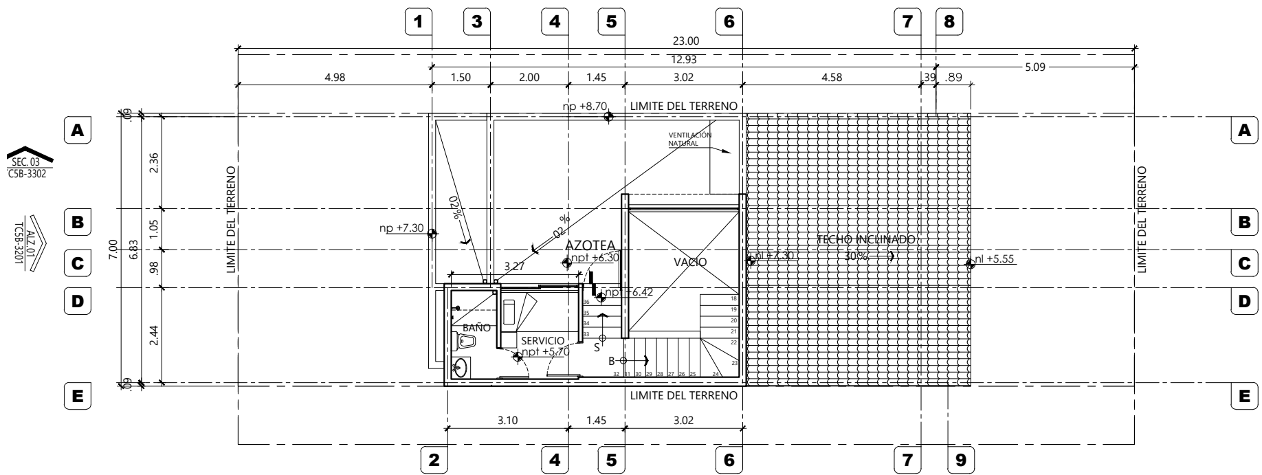
Planta Techos
