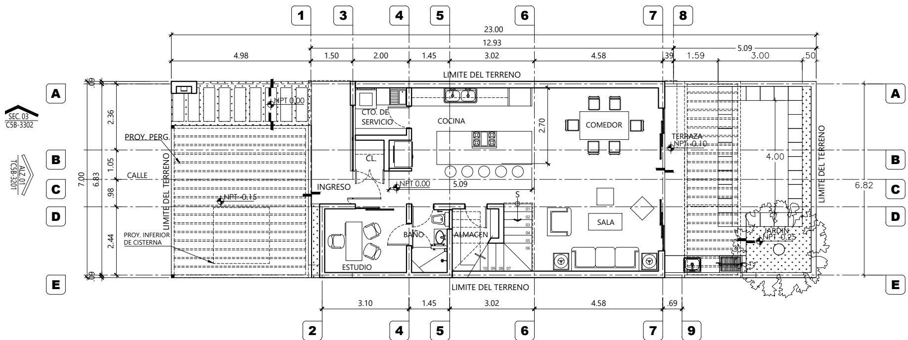
Planta Baja
