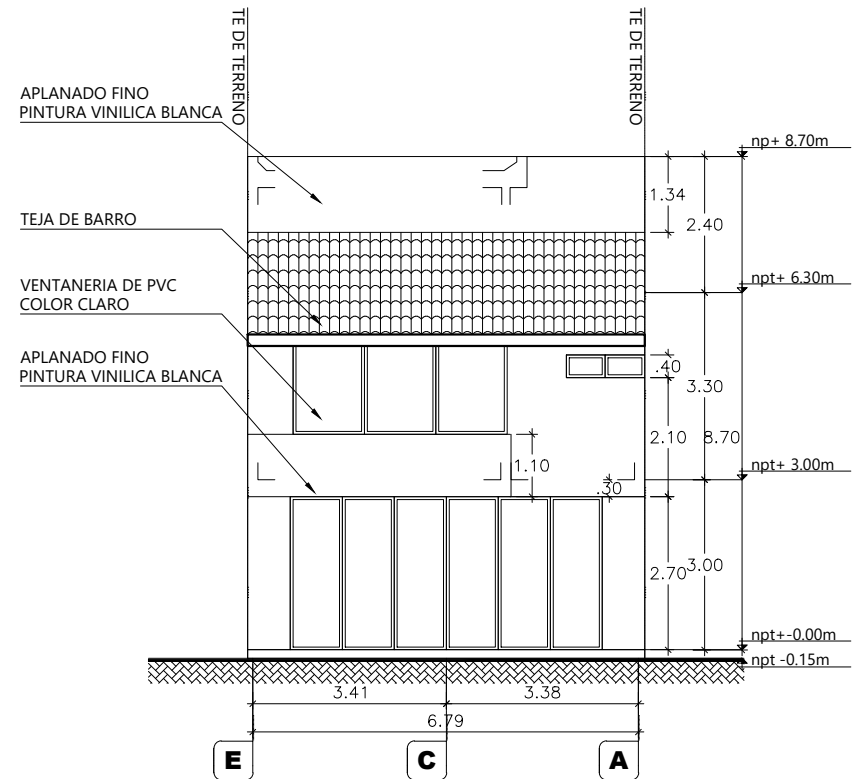
Alzado Posterior
