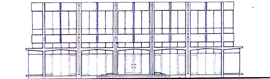
Elevación Norte
