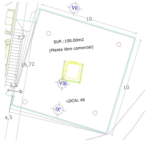
SEGUNDO NIVEL
