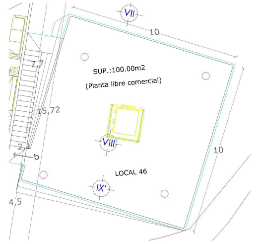
TERCER NIVEL
