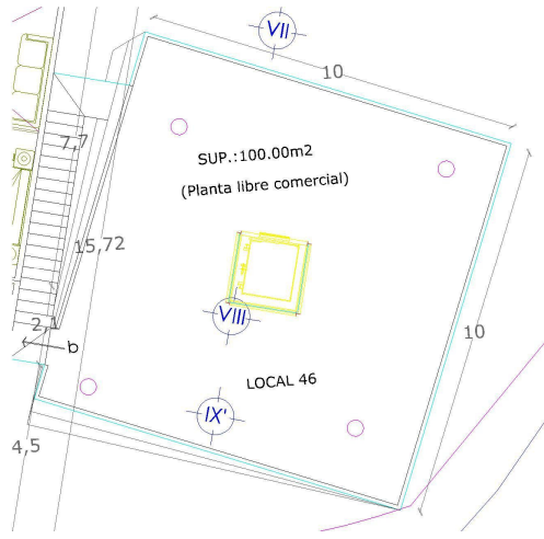
PRIMER NIVEL
