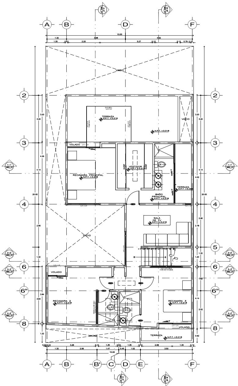
Planta Alta
