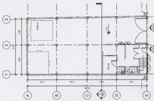
01 Planta Baja 1:100
