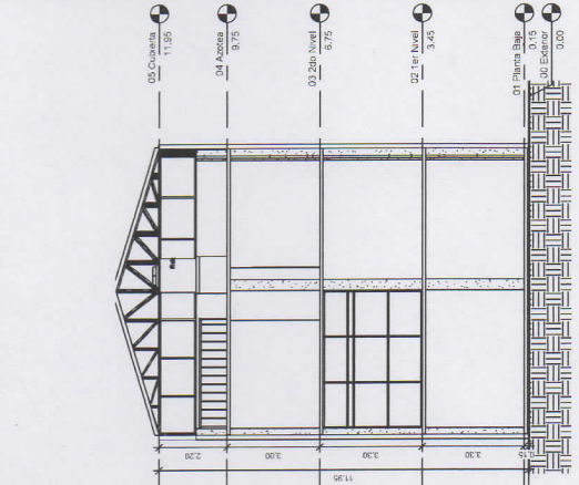
03 Sección 1 1:75
