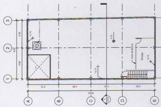
04 Azotea 1:100
