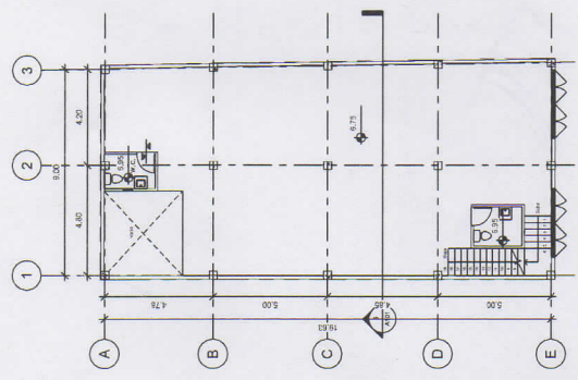
03 2do Nivel 1:100
