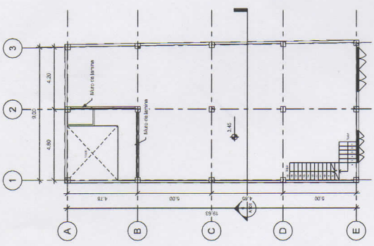
02 1er Nivel 1:100
