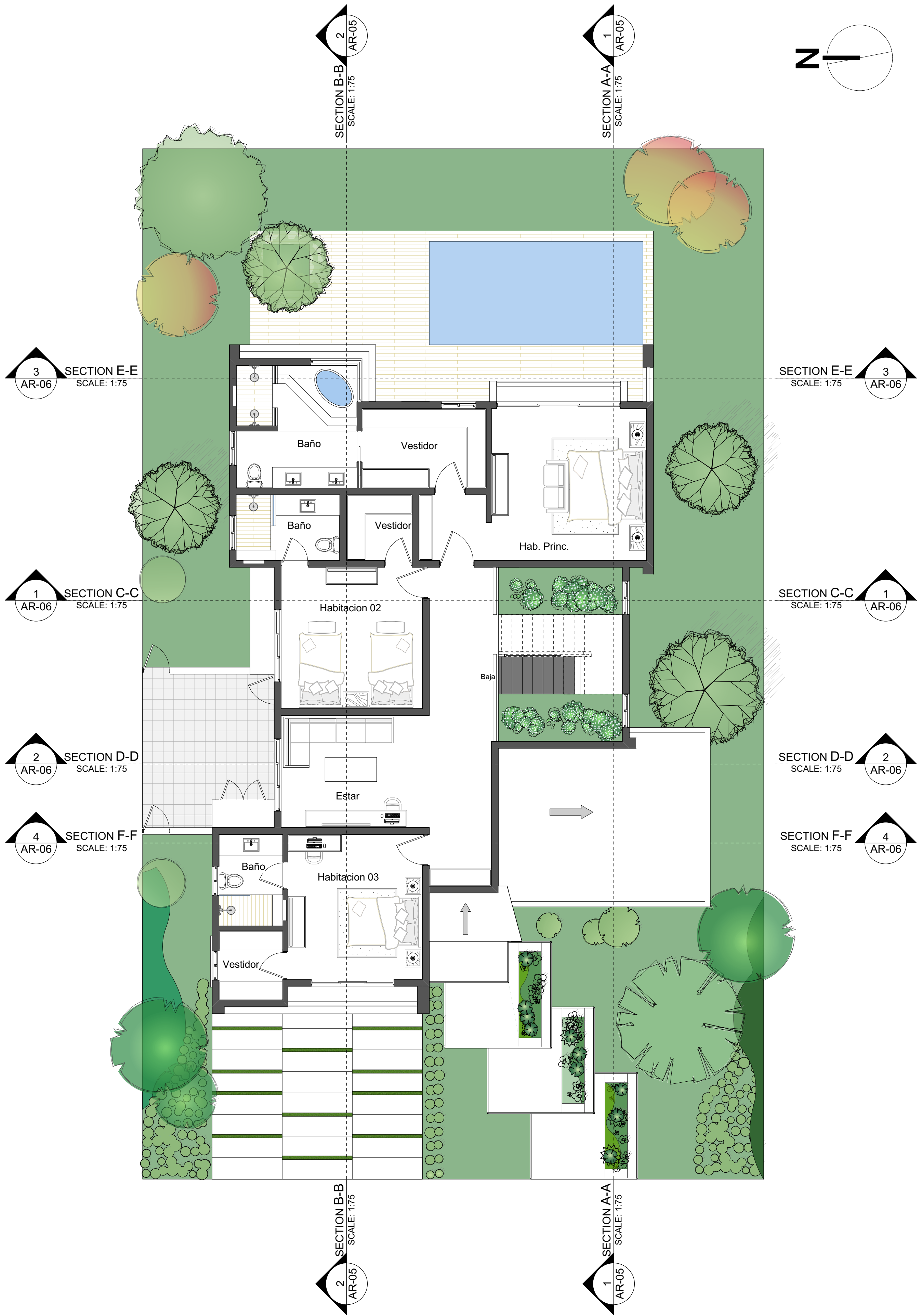
2 PLANTA ARQUITECTONICA 2DO NIVEL Scale: 1:75
