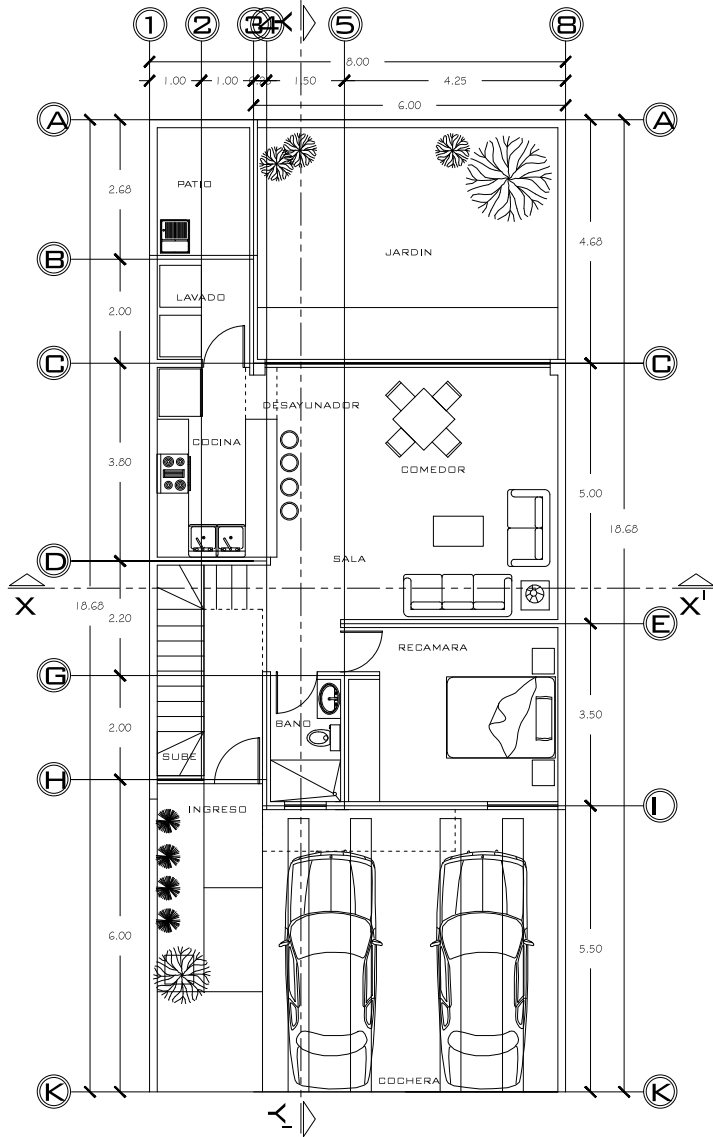
P LANTA ARQUITECTONICA BAJA ESCALA 1 : 100 / 77.00 M2 CONST
