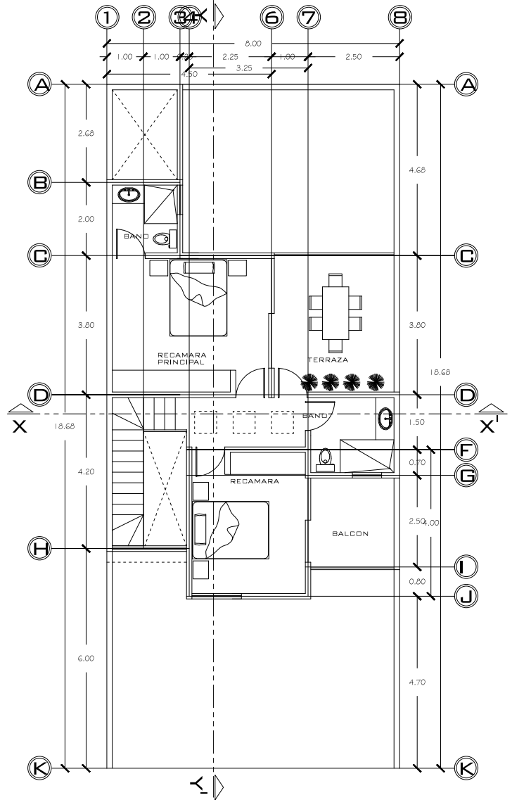
P LANTA ARQUITECTONICA ALTA ESCALA 1 : 100 / 58.00 M2 CONST
