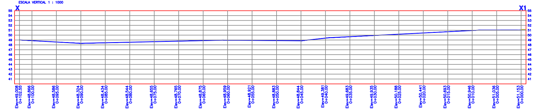
PERFIL LONGITUDINAL ESCALA HORIZONTAL 1 : 1000 ESCALA VERTICAL 1 : 1000
