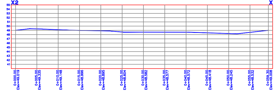
PERFIL TRANSVERSAL ESCALA HORIZONTAL 1 : 1000 ESCALA VERTICAL 1 : 1000
