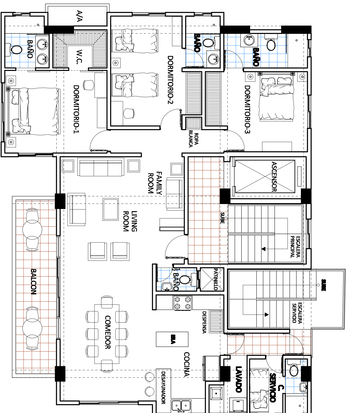
PLANTA ARQUITECTONICA 3er al 6to NIVEL TORRE YELO-1
