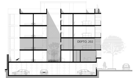
CORTE TRANSVERSAL
