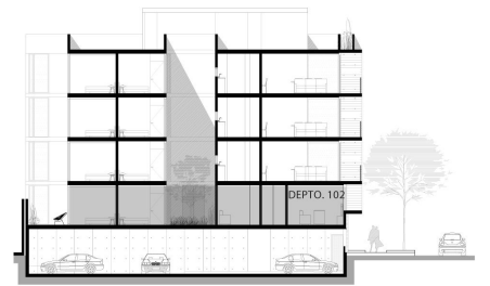
CORTE TRANSVERSAL
