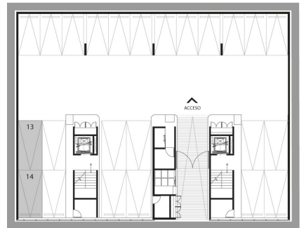
ESTACIONAMIENTO
