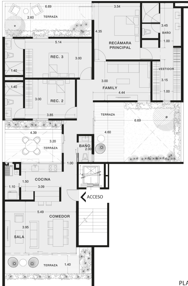
PLANTA
