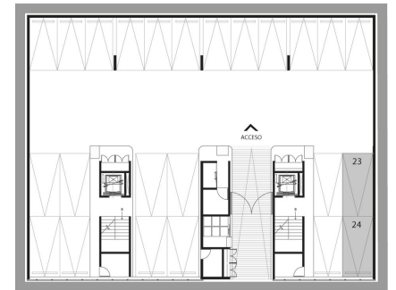
ESTACIONAMIENTO
