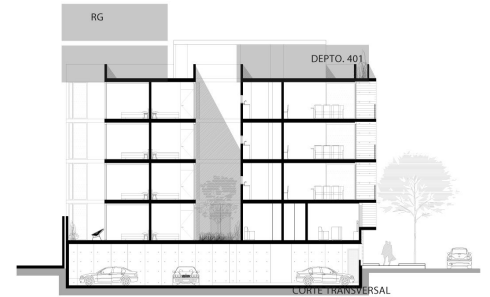
CORTE TRANSVERSAL
