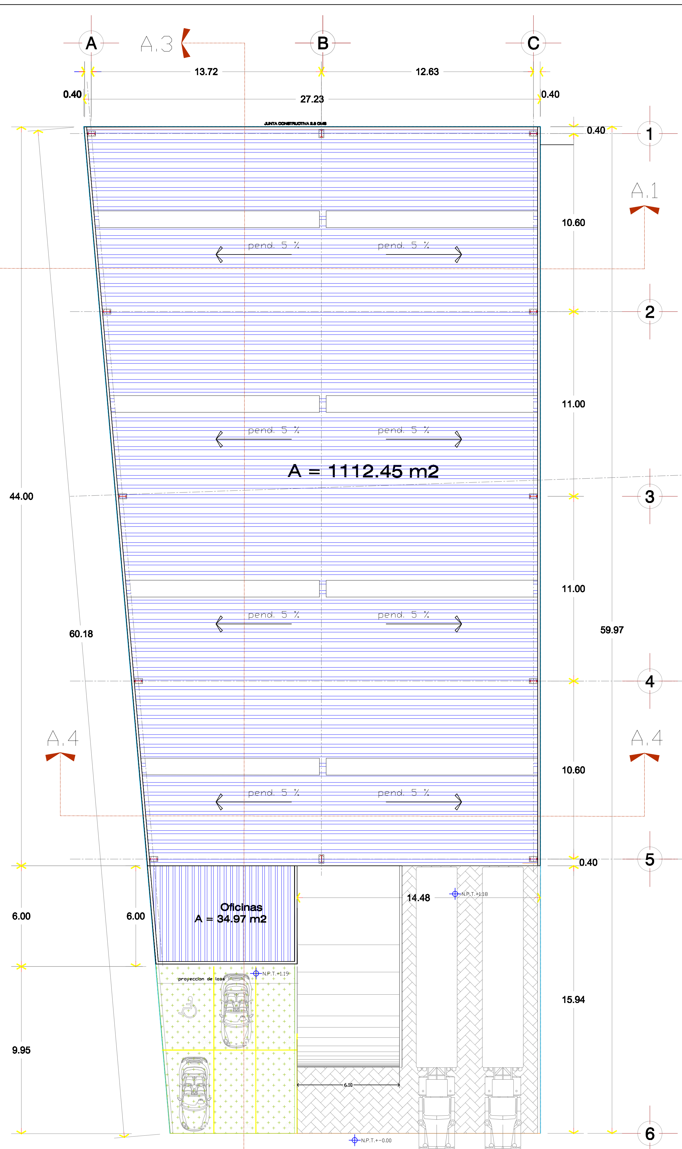
PLANTA DE CONJUNTO ESC. 1:125
