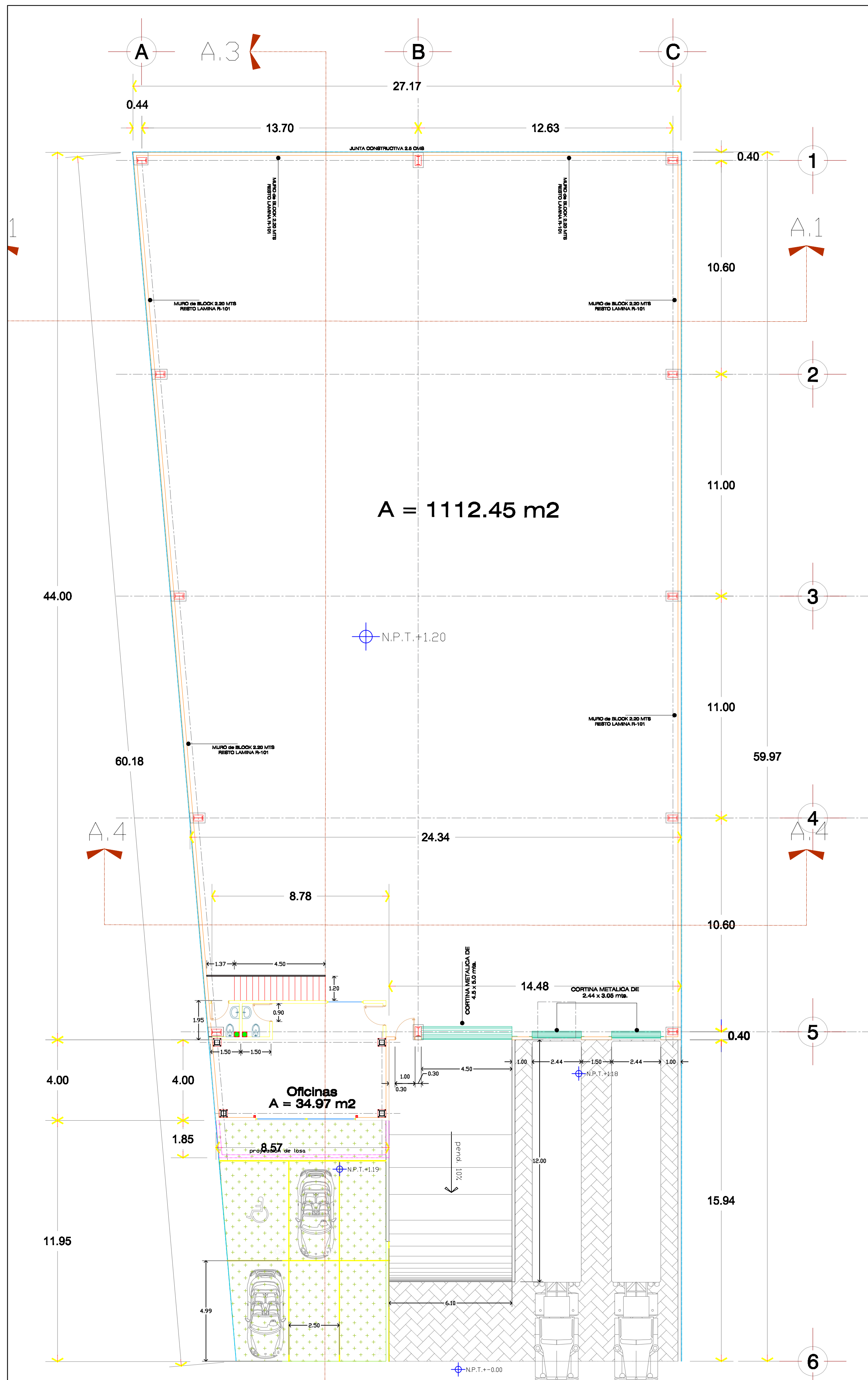
PLANTA ARQUITECTONICA ESC. 1:125
