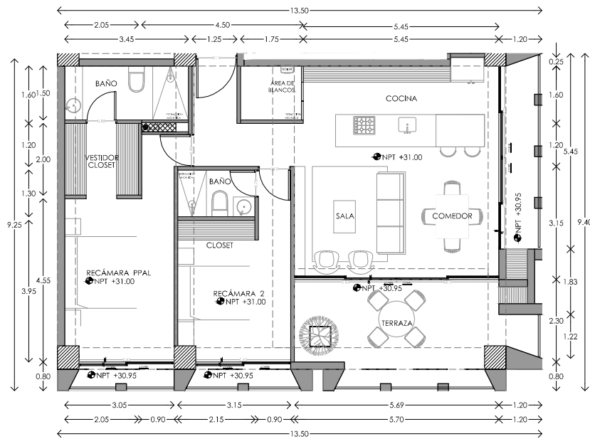
DEPARTAMENTO 902 ESCALA 1:150
