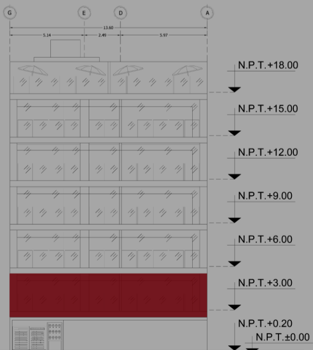
FACHADA POSTERIOR CALLE ALICAMA
