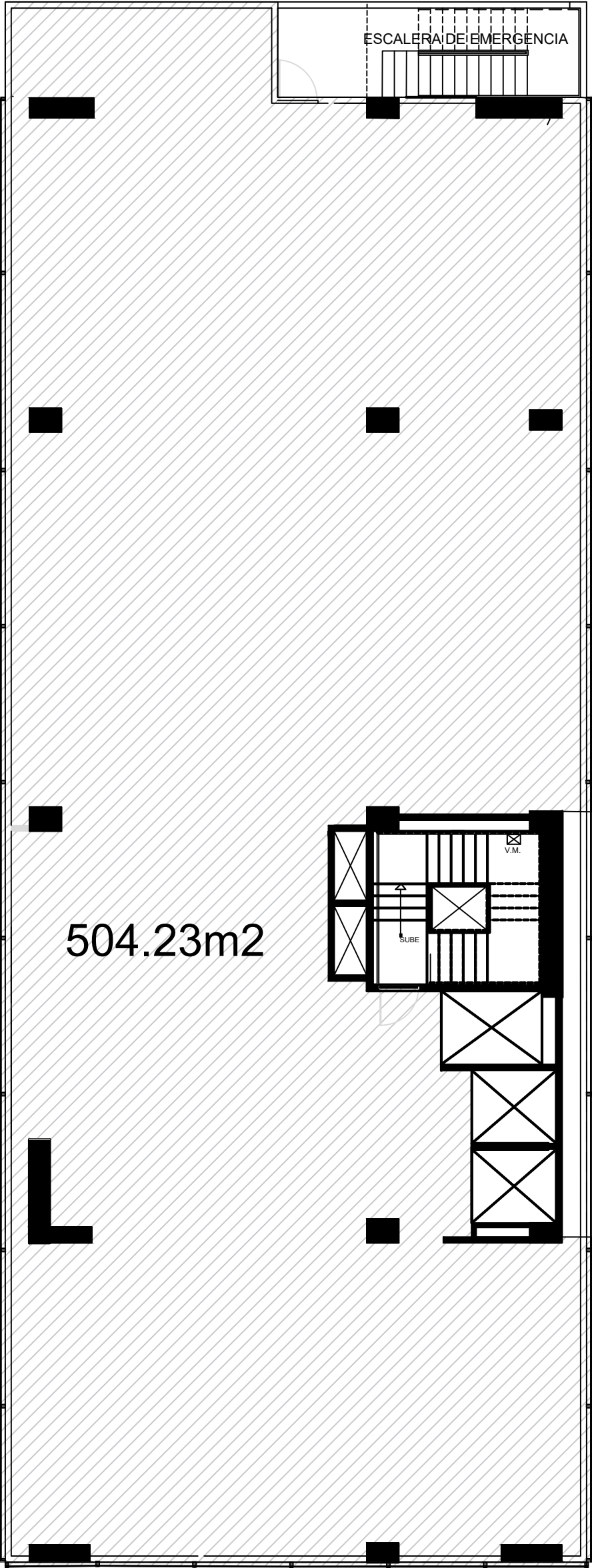
PLANTA LIBRE 504.23m2
