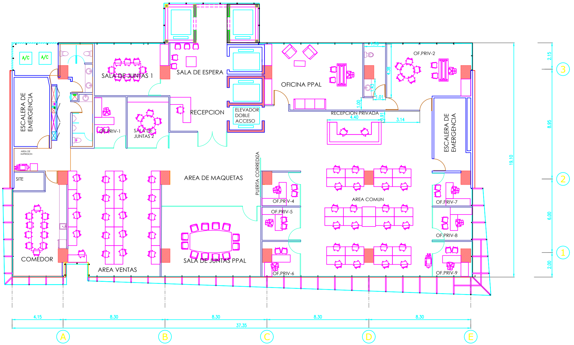
PLANTA ARQUITECTONICA
