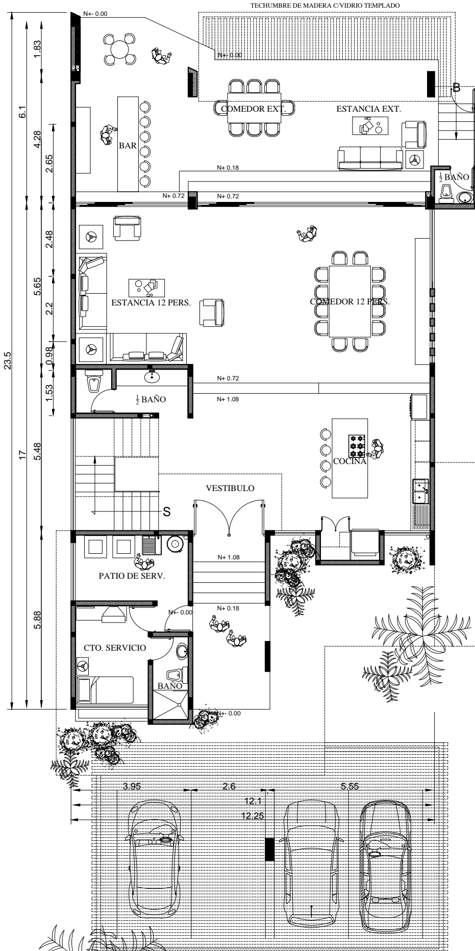
ARQ. PLANTA BAJA VILLA 12
