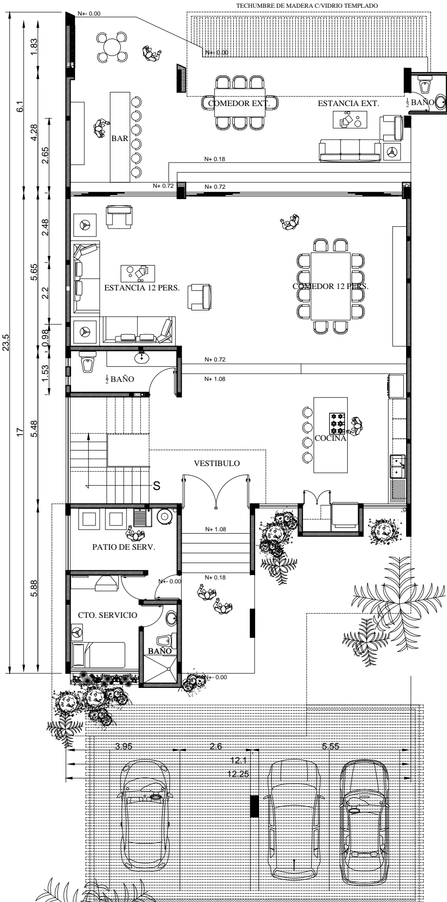
ARQ. PLANTA BAJA VILLA 7 -11
