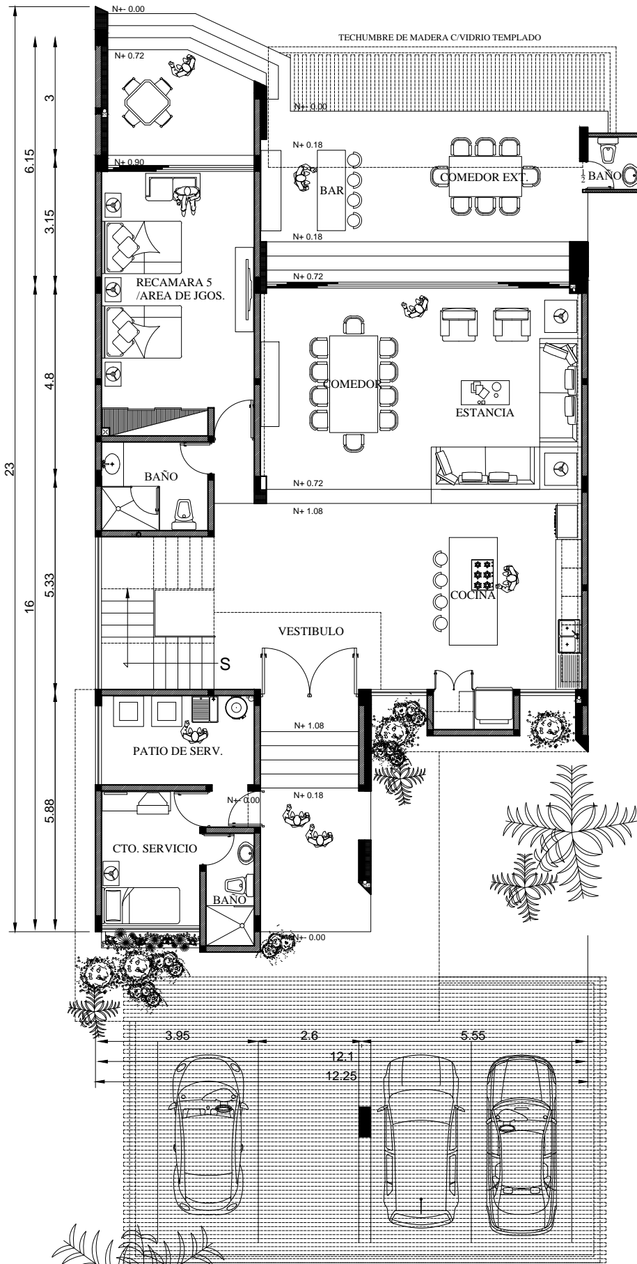
ARQ. PLANTA BAJA VILLA 1 - 6
