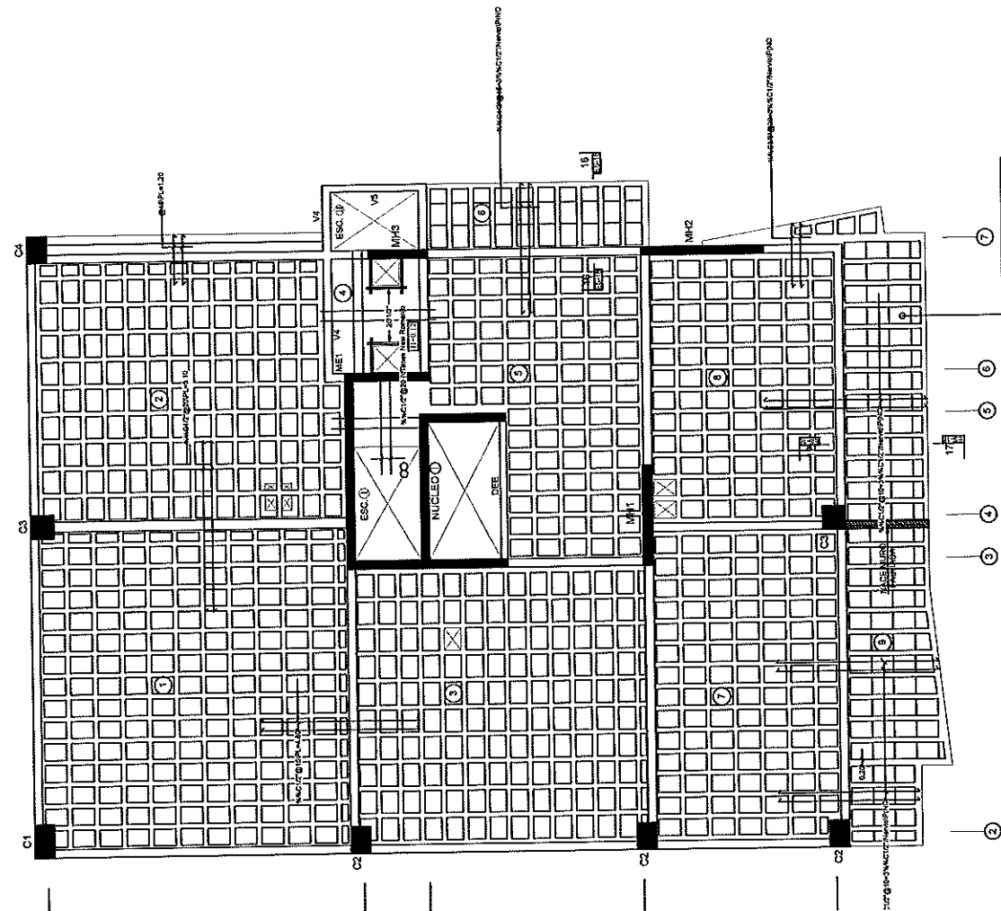
SISTEMA Y DIMENSIONES 12VO. NIVEL Esc: 1:200
