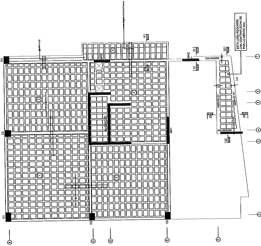
SISTEMA Y DIMENSIONES TECHO Esc: 1:200
