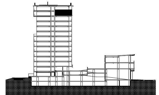
CORTE ESQUEMATICO
