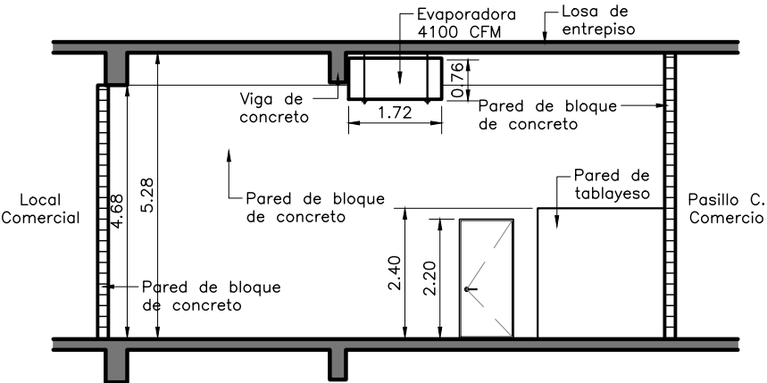
SECCIÓN B-B
