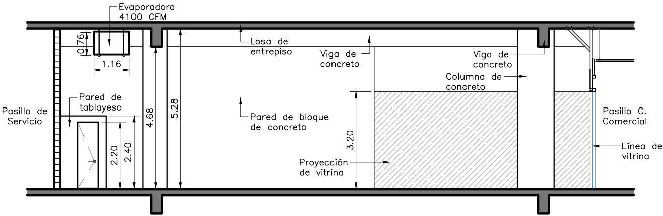
SECCIÓN A-A
