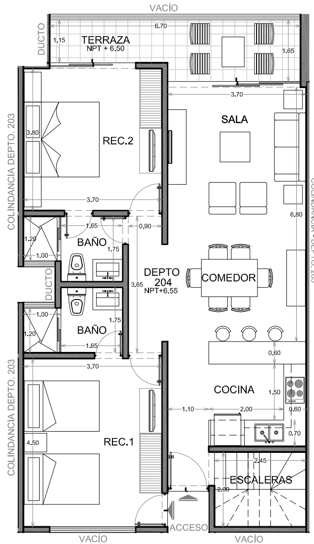
PLANTA ARQUITECTÓNICA ESC. 1:100
