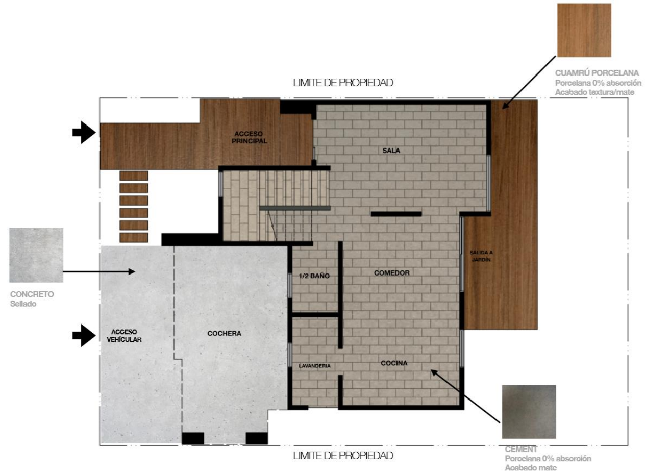
Planta Baja
