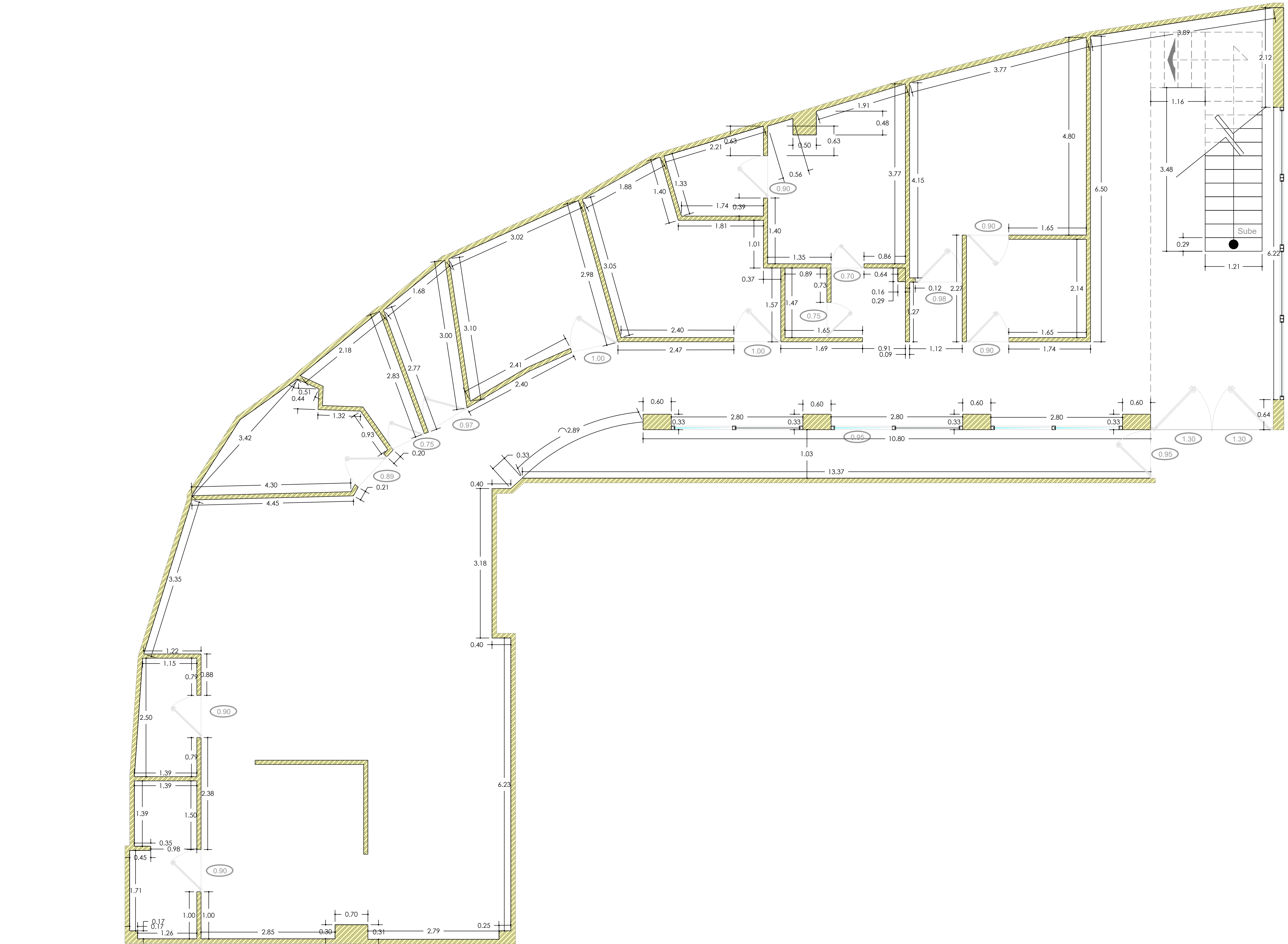
PLANTA BAJA ESC. 1:40
