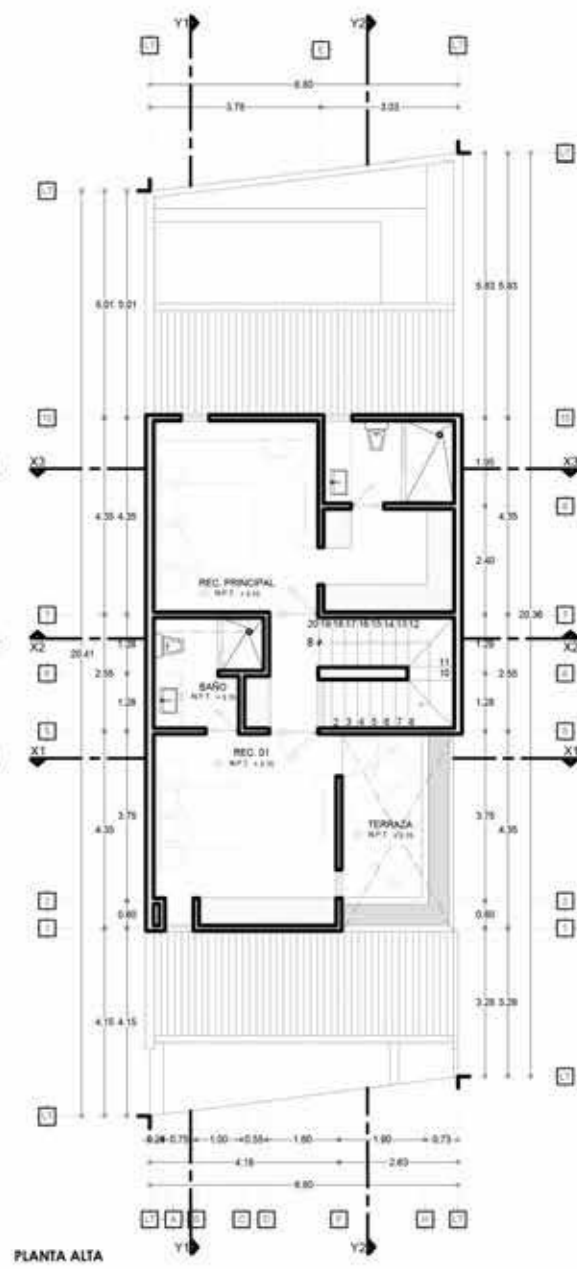
PLANTA ALTA
