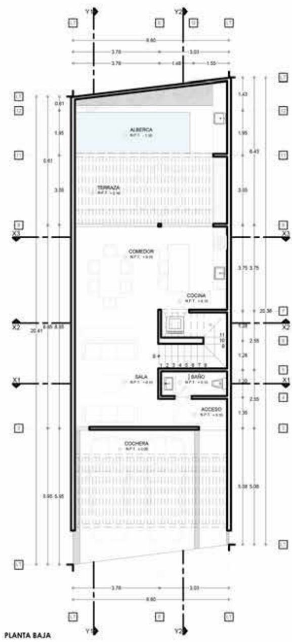
PLANTA BAJA
