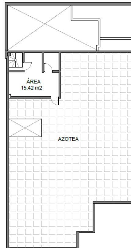
PLANTA AZOTEA
