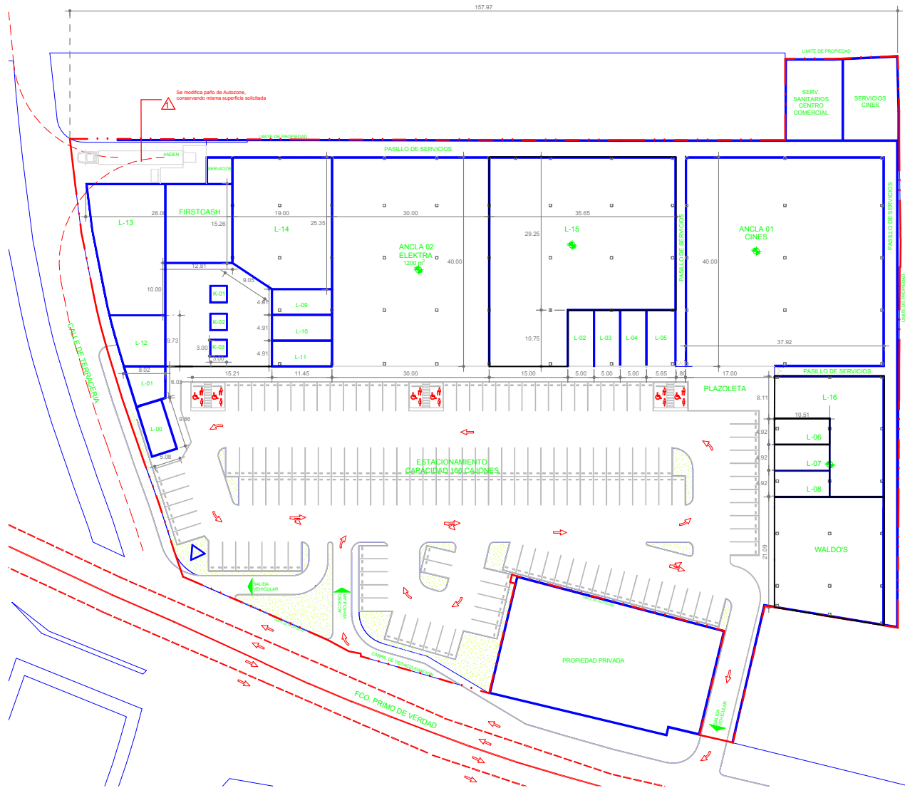
A1 PLANTA BAJA ARQUITECTÓNICA 1 : 400
