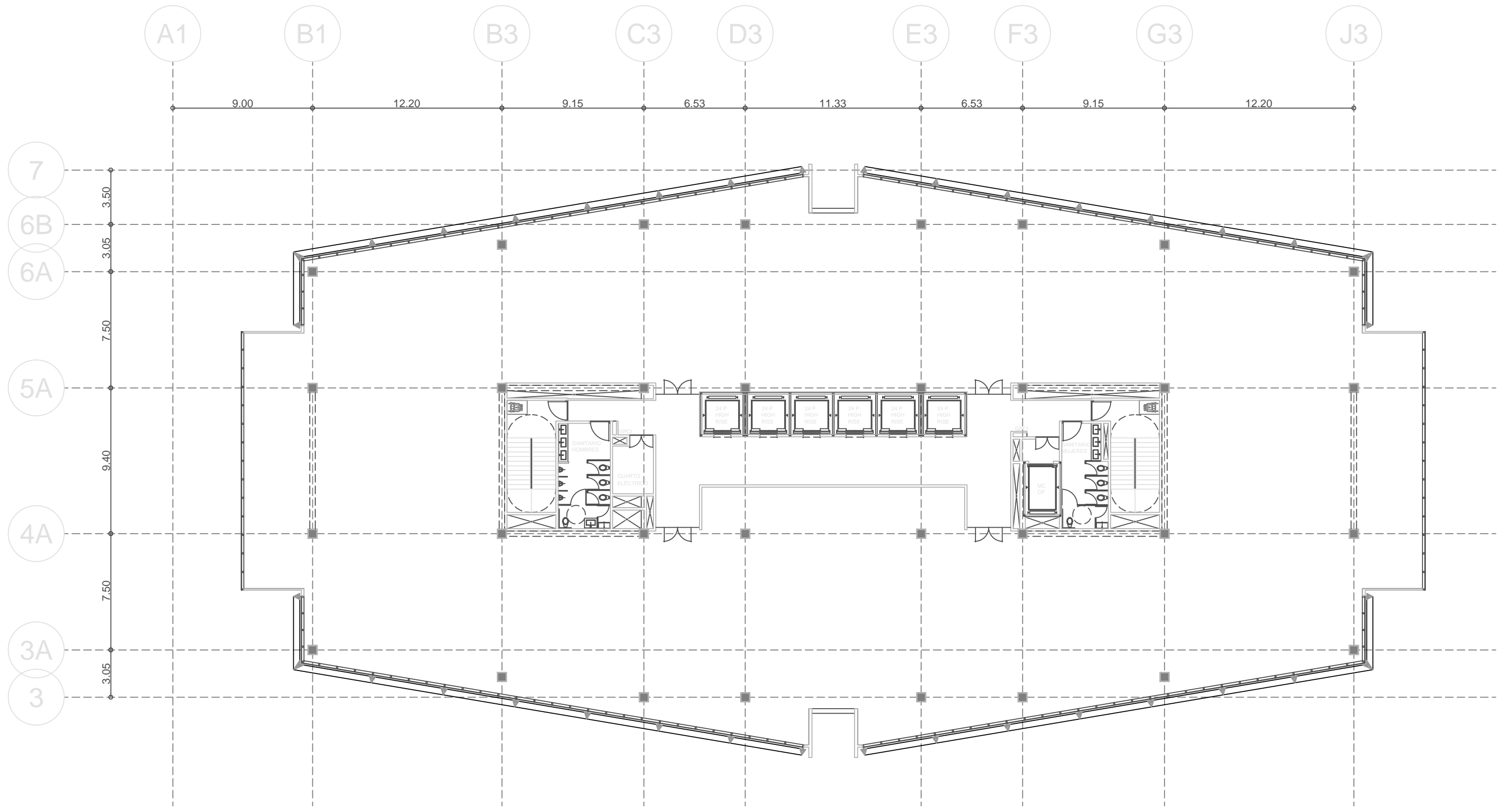
PLANTA TIPO HIGH RISE
