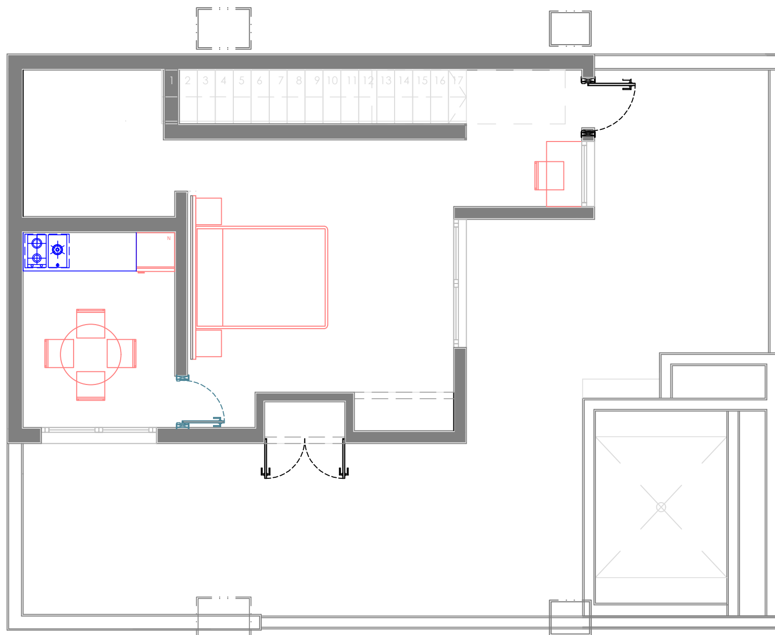
PLANTA ARQUITECTONICA D5 (PENTHOUSE)
