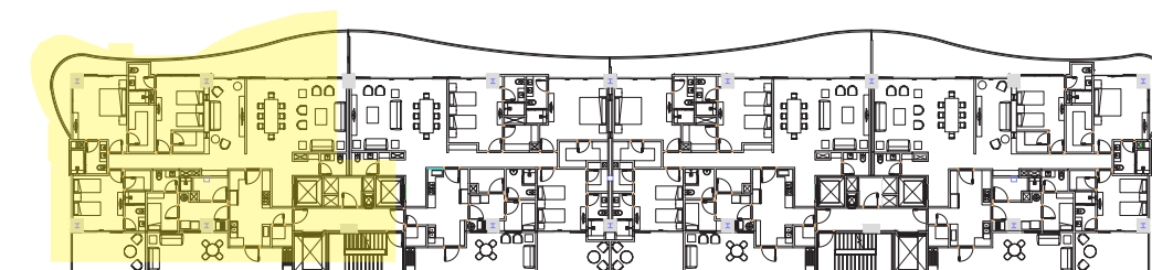
PLANTA ESQUEMÁTICA NIVEL 2
