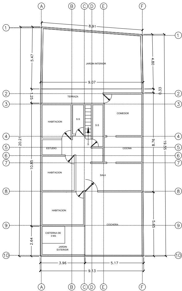
PLANTA ARQUITECTONICA PRIMER NIVEL
