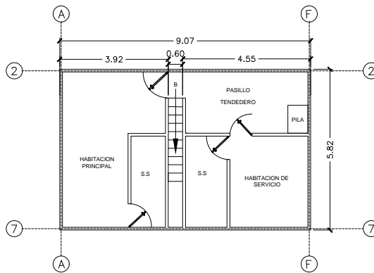
PLANTA ARQUITECTONICA SEGUNDO NIVEL
